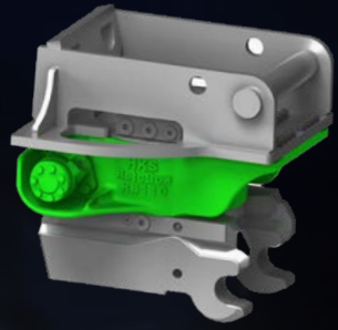
DREHBARER SCHNELLWECHSLER
